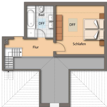
Grundriss Schlafen
