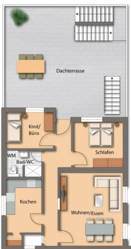
Grundriss
