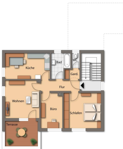
Grundriss
