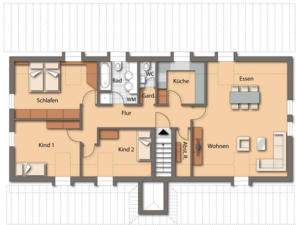
Grundriss 3. OG
